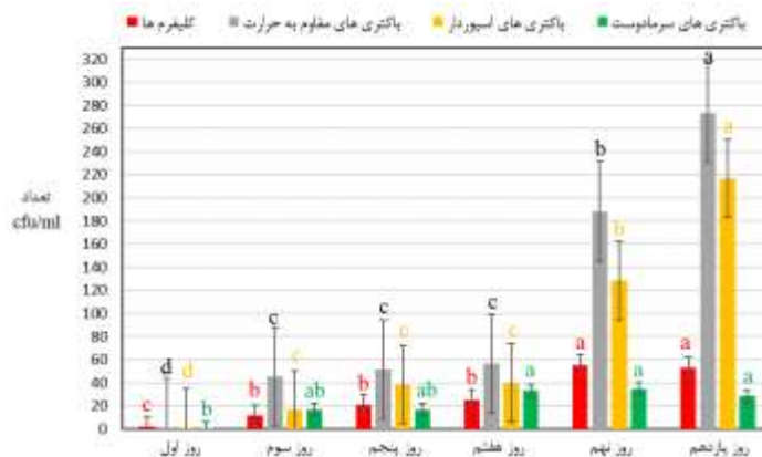
نمودار ۵- اثر زمان در دمای ۱۵ درجه سلسیوس بر تعداد کلی فرم‌ها، باکتری‌های مقاوم به حرارت، باکتری‌های اسپوردان و باکتری‌های سرمادوست در خامه پاستوریزه
