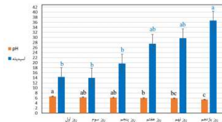
نمودار ۶- اثر زمان در دمای ۱۵ درجه سلسیوس بر میزان pH و اسیدیته خامه پاستوریزه
