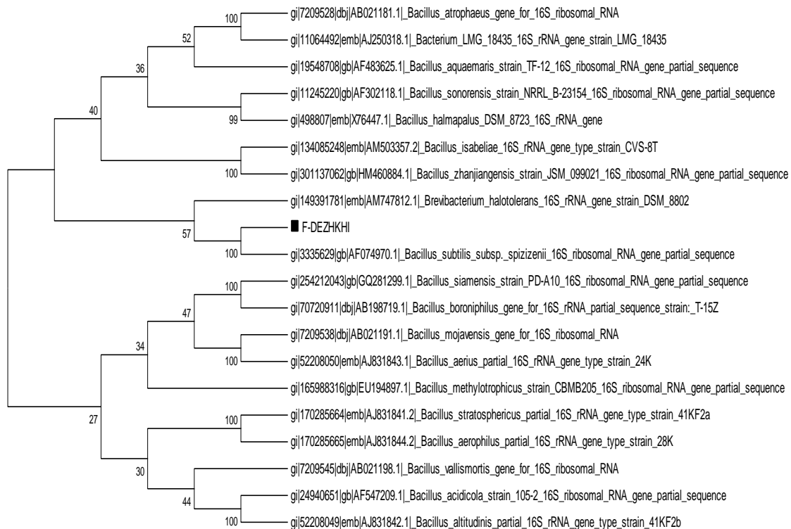
شکل ۳- درخت فیلوژنتیکی ترسیم شده برای جدایه باکتری F و وضعیت تاکسونومیکی آن
