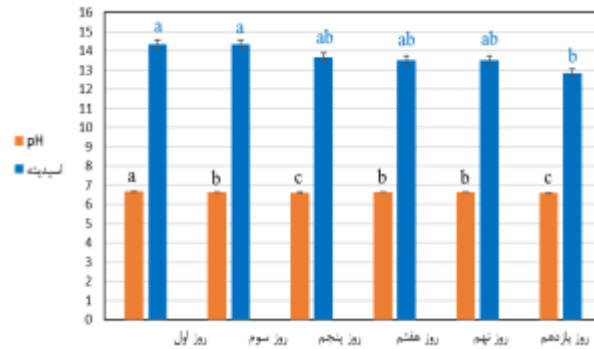
نمودار ۳- اثر زمان در دمای ۴ درجه سلسیوس بر میزان pH و اسیدیته خامه پاستوریزه
